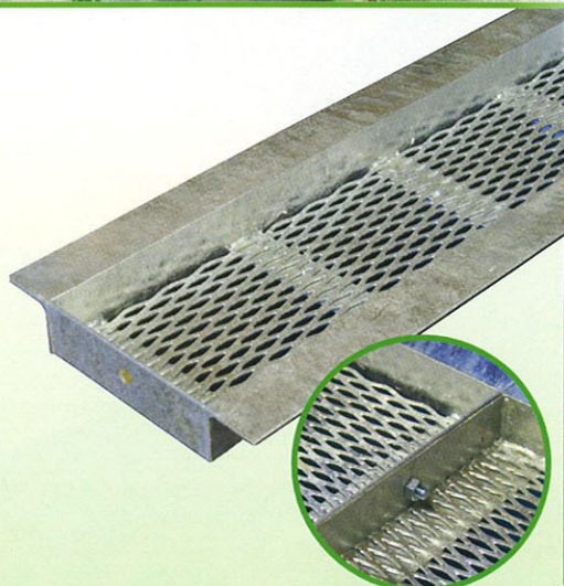
連結例 (M8ボルト・ナット別途)
